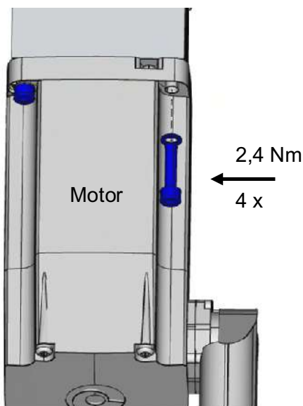
Abbildung 2 Montage Motor
