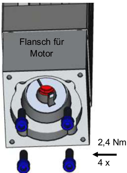
Abbildung 2 Montage Flansch
