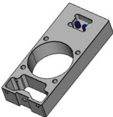
Abbildung 3 Montagerahmen
