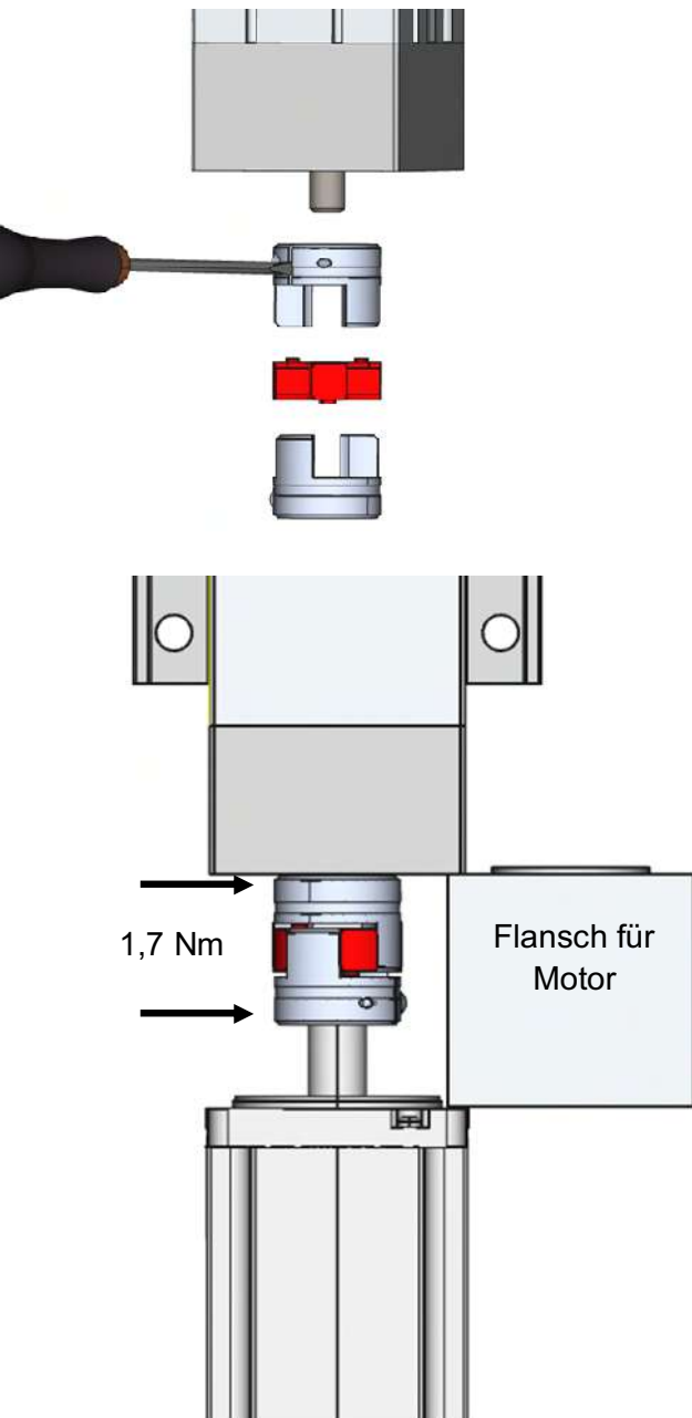
Abbildung 1 Montage
