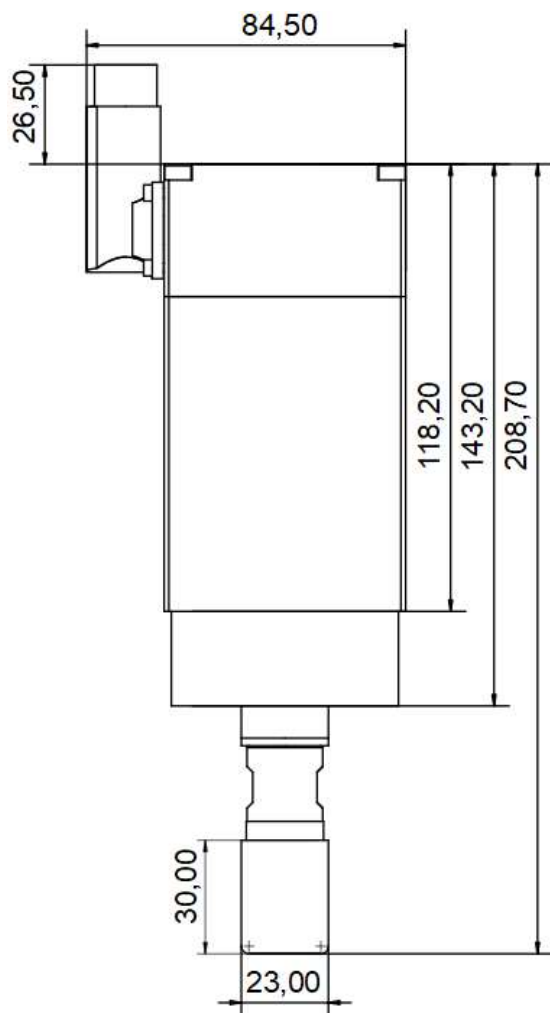
Compact Modul mit Wechseladapter
